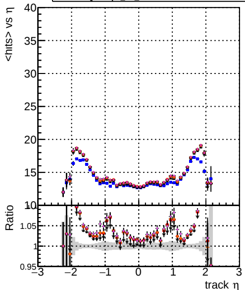
DOMstep3 CKF DOMstep3 default DOMstep3 CKPixelLess DOMstep3 default-refl2 DOMstep3 defaultNEWTOLDSAMPLE-refl2
