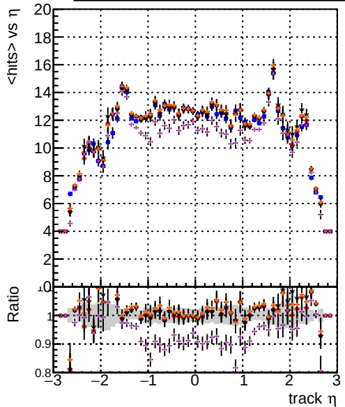
mean hits DOMstep3 TT CKF DOMstep3 TT default DOMstep3 TT ckfPixelLess DOMstep3 TT default-refl2 DOMstep3 TT defaultNEWTOLDSAMPLE-refl2
