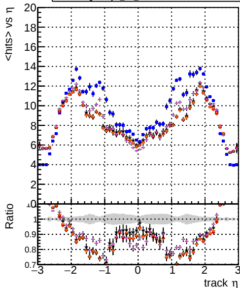
DOMstep3 TT CKF DOMstep3 TT default DOMstep3 TT ckPixelLess DOMstep3 TT default-ref12 DOMstep3 TT defaultNEWTOLDSAMPLE-ref12 mean hit
