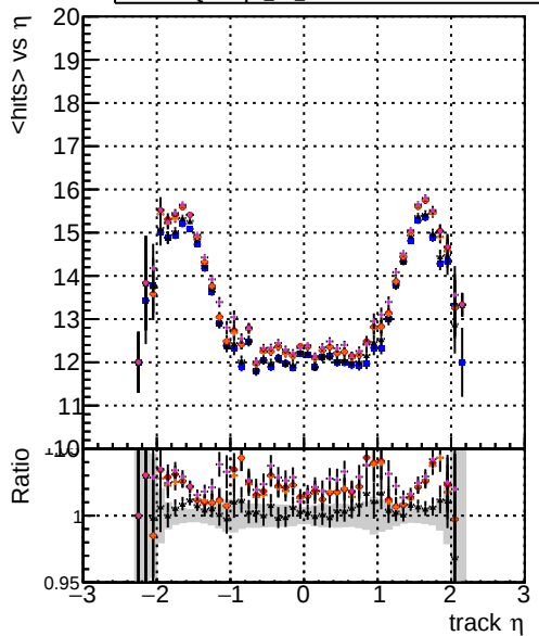
mean hits vs \eta DOMstep3 CKF DOMstep3 default DOMstep3 CKPixelLess DOMstep3 default-ref DOMstep3 defaultNEWTOLDSAMPLE-ref
