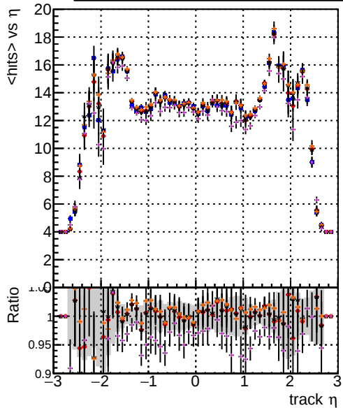
mean hit DOMstep3 CKF DOMstep3 default DOMstep3 CKFPixelLess DOMstep3 default-ref DOMstep3 default-NEWTOLDSAMPLE-ref
