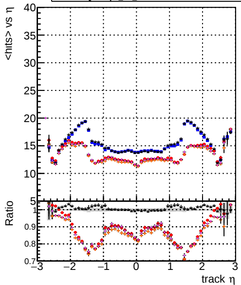
mean hits vs \eta DOMstep3 TT CKF DOMstep3 TT default DOMstep3 TT ckPixelLess DOMstep3 TT default-refl DOMstep3 TT defaultNEWTOLDSAMPLE-refl
