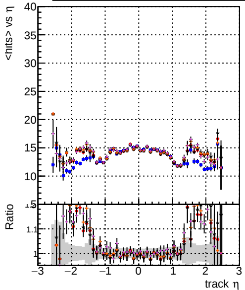
mean hits DOMstep3 CKF default DOMstep3 CKFPixelLess DOMstep3 default-ref DOMstep3 default-NEWTOLDSAMPLE-ref
