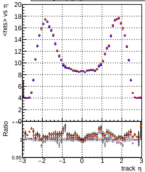
DOMstep3 CKF DOMstep3 default DOMstep3 ckPixelLess DOMstep3 default-ref DOMstep3 defaultNEWTOLDSAMPLE-ref
