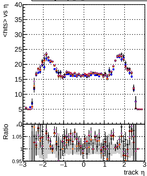
mean hit DOMstep3 CKF DOMstep3 ckPixelLess DOMstep3 default DOMstep3 default+relf DOMstep3 default+NEWTOLDSAMPLE+relf
