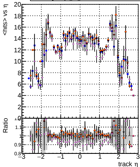
mean hits DOMstep3 TT CKF DOMstep3 TT default DOMstep3 TT CKPixelLess DOMstep3 TT default-ref DOMstep3 TT defaultNEWTOLDSAMPLE-ref
