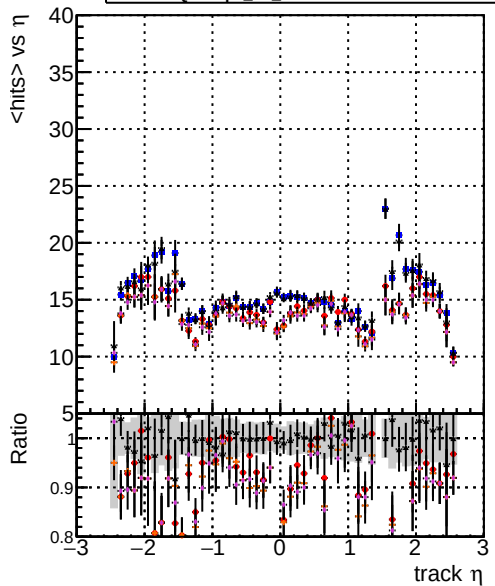
mean hits vs \eta DOMstep3 TT CKF DOMstep3 TT default DOMstep3 TT ckrPixelLess DOMstep3 TT default-ref DOMstep3 TT defaultNEWTOLDSAMPLE-ref
