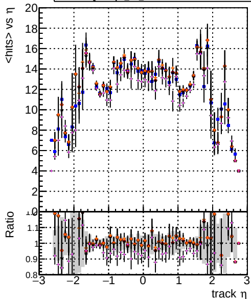
mean hit DOMstep3 TT CKF DOMstep3 TT default DOMstep3 TT ckrPixelLess DOMstep3 TT default-refl DOMstep3 TT defaultNEWTOLDSAMPLE-refl
