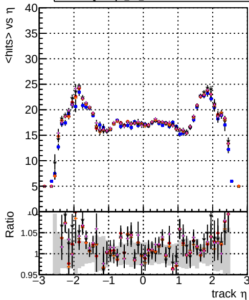
DOMstep3 TT CKF DOMstep3 TT default DOMstep3 TT CKFPixelLess DOMstep3 TT default-ref DOMstep3 TT defaultNEWTOLDSAMPLE-ref
