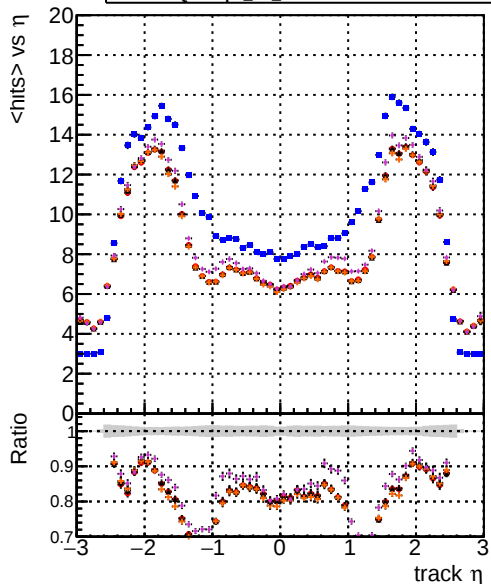
mean hits DOMstep3 TT CKF DOMstep3 TT default DOMstep3 TT CKPixelLess DOMstep3 TT default-ref DOMstep3 TT defaultNEWTOLDSAMPLE-ref
