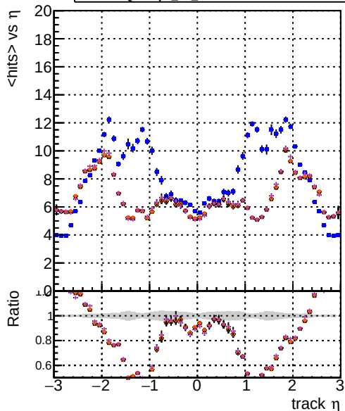
mean hit DOMstep3 TT default CKF DOMstep3 TT default ckrPixelLess DOMstep3 TT default-ref DOMstep3 TT defaultNEWTOLDSAMPLE-ref
