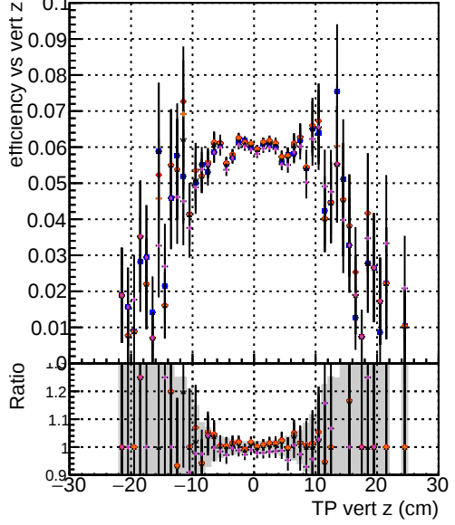
Efficiency vs. TP vert z (cm) DOMstep3 CKF DOMstep3 default DOMstep3 ckrPixelLess DOMstep3 default-ref DOMstep3 defaultNEWTOLDSAMPLE-ref
