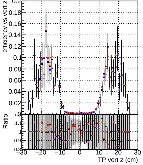
Efficiency vs. sim PV z DOMstep3 ckf DOMstep3 default DOMstep3 ckfPixelLess DOMstep3 default-refl DOMstep3 defaultNEWTOLDSAMPLE-refl
