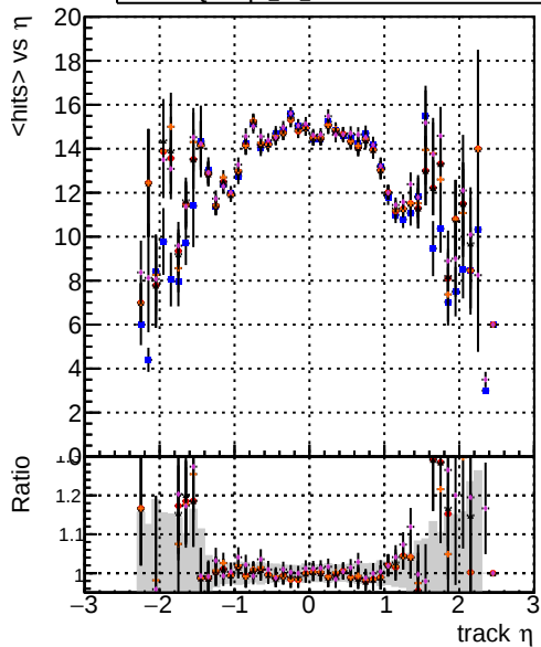
mean hits vs \eta DOMstep3 TT CKF DOMstep3 TT default DOMstep3 TT CKPixelLess DOMstep3 TT default-ref DOMstep3 TT defaultNEWTOLDSAMPLE-ref
