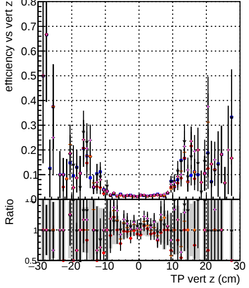
Efficiency vs. TP vert z Legend: DOMstep3 CKF DOMstep3 default DOMstep3 ckPixelLess DOMstep3 default-refl DOMstep3 defaultNEWTOLDSAMPLE-refl
