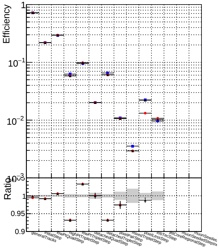
DQMstep3_SoftQCD_CKF DQMstep3_SoftQCD_default DQMstep3_SoftQCD_ckfPixelLess
