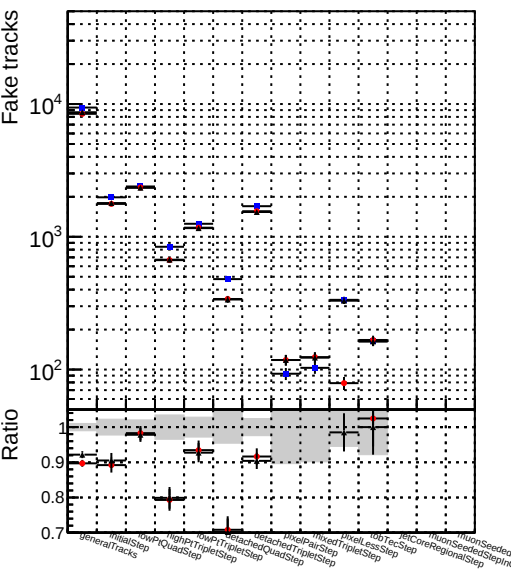
Number Legend DQMstep3_SoftQCD_default DQMstep3_SoftQCD_ckfPixelLess
