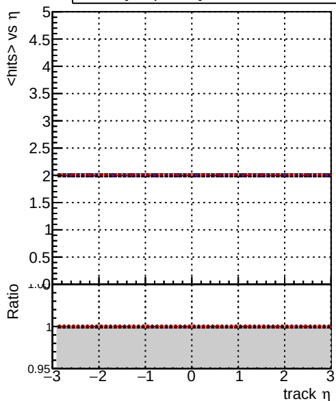
mean hits DQMstep3_SoftQCD_CKF DQMstep3_SoftQCD_default DQMstep3_SoftQCD_ckfPixelLess
