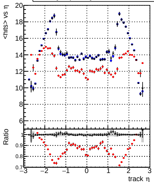
mean hits — DQMstep3_SoftQCD_CKF — DQMstep3_SoftQCD_default — DQMstep3_SoftQCD_ckfPixelLess
