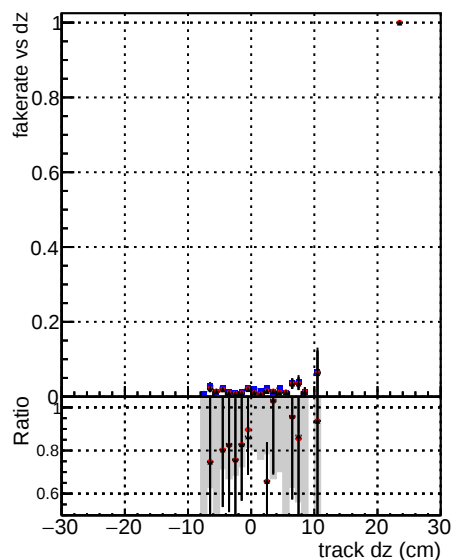
DOMstep3 SoftOCD-CKF DOMstep3 SoftOCD default DOMstep3 SoftOCD-CKF PixelLess
