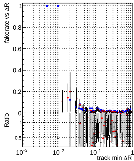
—•— DQMstep3_SoftQCD_CKF —•— DQMstep3_SoftQCD_default —•— DQMstep3_SoftQCD_ckfPixelLess
