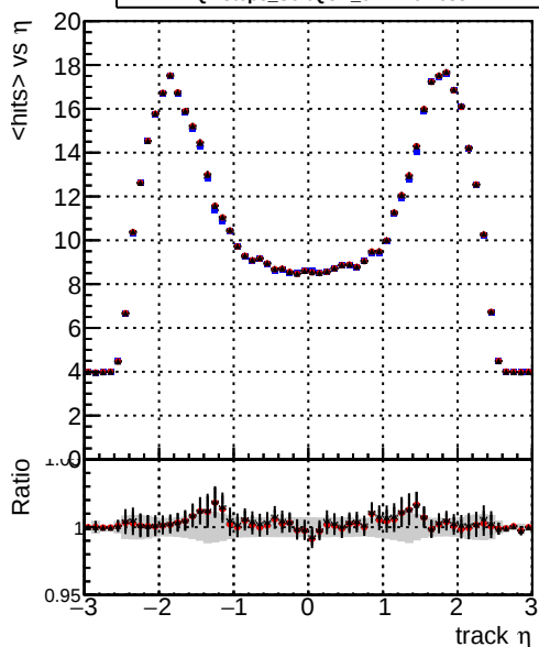
mean hits vs \eta DQMstep3_SoftQCD_CKF DQMstep3_SoftQCD_default DQMstep3_SoftQCD_ckfPixelLess
