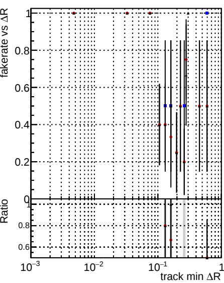
Legend: DQMstep3_SoftQCD_CKF (grey squares), DQMstep3_SoftQCD_default (red circles), DQMstep3_SoftQCD_ckfPileLess (black triangles)
