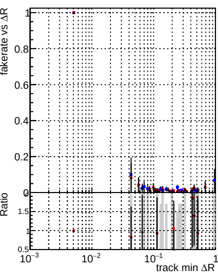
Legend: DQMstep3_SoftQCD_CKF (grey bars), DQMstep3_SoftQCD_default (blue dots), DQMstep3_SoftQCD_ckfPileLess (red dots)
