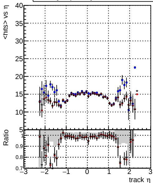
mean hits vs \eta — DQMstep3_SoftQCD_CKF — DQMstep3_SoftQCD_default — DQMstep3_SoftQCD_ckfPixelLess
