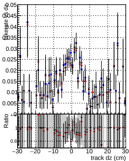
—•— DOMstep3 SoftOCD-CKF —•— DOMstep3 SoftOCD-default —•— DOMstep3 SoftOCD-CKF-PixelLess
