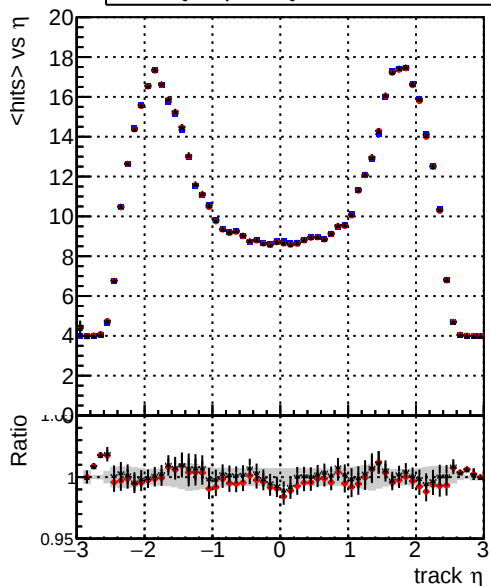
DQMstep3_SoftQCD_CKF DQMstep3_SoftQCD_default DQMstep3_SoftQCD_ckfPixelLess mean hits
