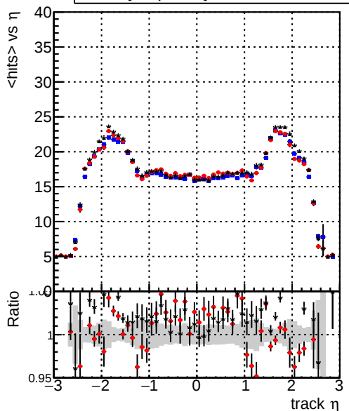
mean hit — DQMstep3_SoftQCD_CKF — DQMstep3_SoftQCD_default — DQMstep3_SoftQCD_ckfPixelLess
