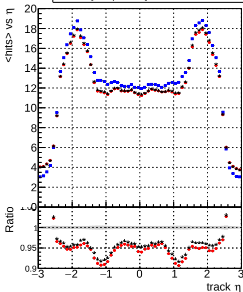
— DQMstep3_SoftQCD_CKF — DQMstep3_SoftQCD_default — DQMstep3_SoftQCD_ckfPixelLess mean hit
