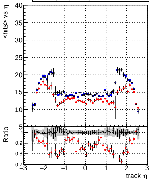
mean hits — DQMstep3_SoftQCD_CKF — DQMstep3_SoftQCD_default — DQMstep3_SoftQCD_ckfPixelLess
