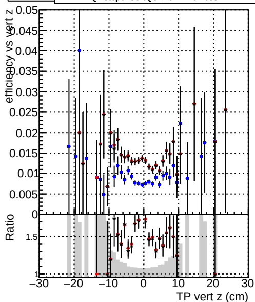
Efficiency vs. sim PV z — DQMstep3_SoftQCD_CKF — DQMstep3_SoftQCD_default — DQMstep3_SoftQCD_ckfPixelLess
