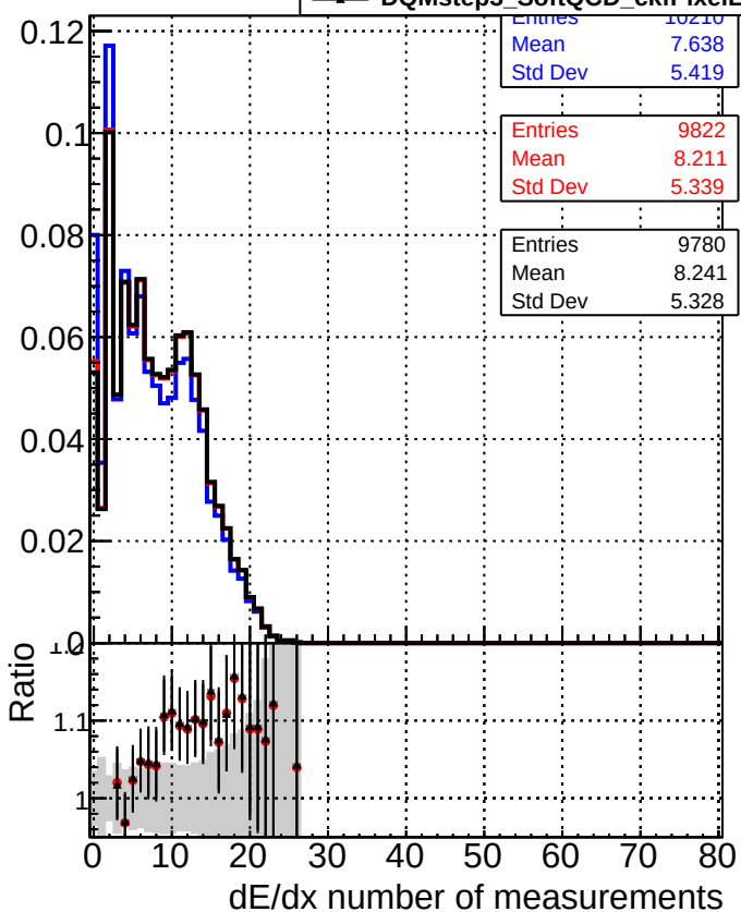
DQMstep3_SoftQCD_CKF DQMstep3_SoftQCD_default DQMstep3_SoftQCD_ckfPixelLess
