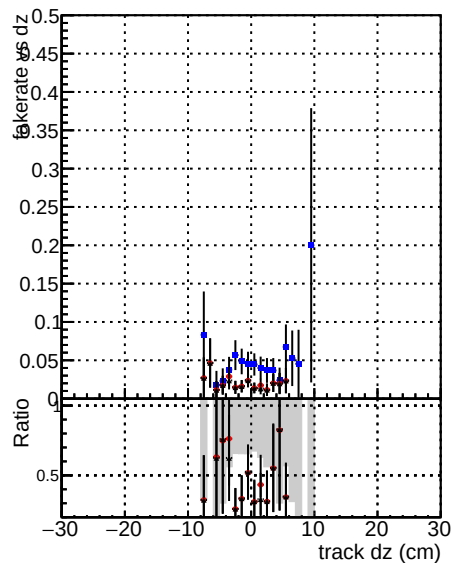
Fake rate vs dz DOMstep3 SoftOCD CKF DOMstep3 SoftOCD default DOMstep3 SoftOCD CKF PixelLess
