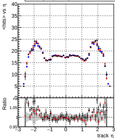
mean hit — DQMstep3_SoftQCD_CKF — DQMstep3_SoftQCD_default — DQMstep3_SoftQCD_ckfPixelLess
