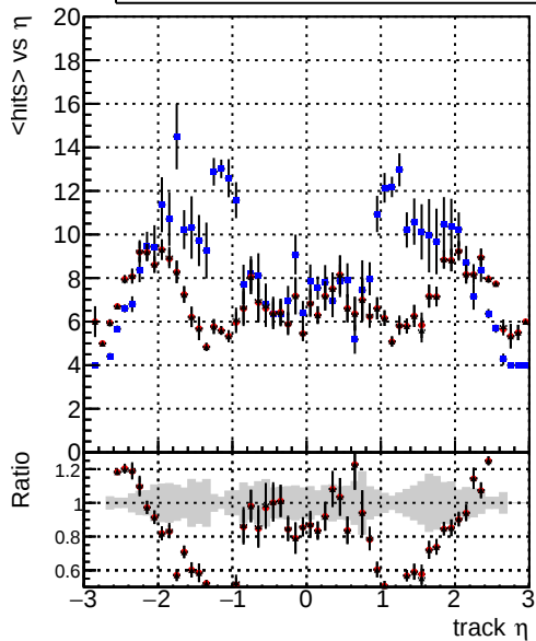
mean hit — DQMstep3_SoftQCD_CKF — DQMstep3_SoftQCD_default — DQMstep3_SoftQCD_ckfPixelLess
