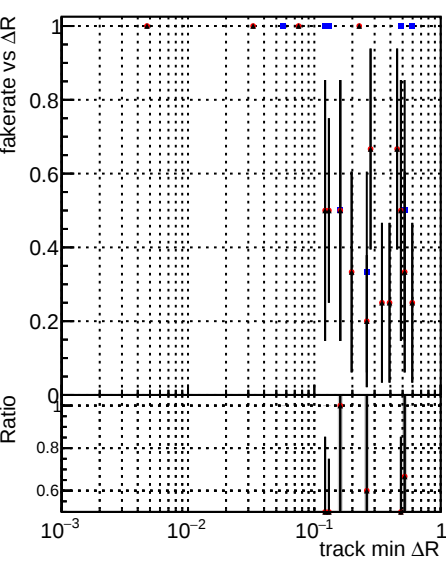
Legend: DQMstep3_SoftQCD_CKF (blue squares), DQMstep3_SoftQCD_default (red circles), DQMstep3_SoftQCD_ckfPileLess (black circles)
