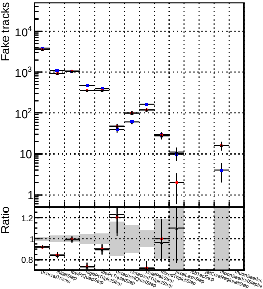
Number DQMstep3_SoftQCD_CKF DQMstep3_SoftQCD_default DQMstep3_SoftQCD_ckfPixelLess
