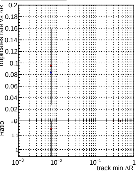
Legend: DQMstep3_SoftQCD_CKF (blue circles), DQMstep3_SoftQCD_default (red circles), DQMstep3_SoftQCD_ckfPixelLess (black circles)
