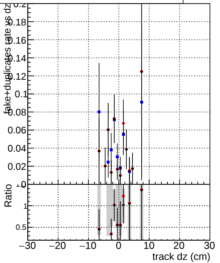
Legend for the plots: DQMstep3_SoftQCD_CKF (Blue squares) DQMstep3_SoftQCD_default (Red circles) DQMstep3_SoftQCD_ckfPixelLess (Black triangles)
