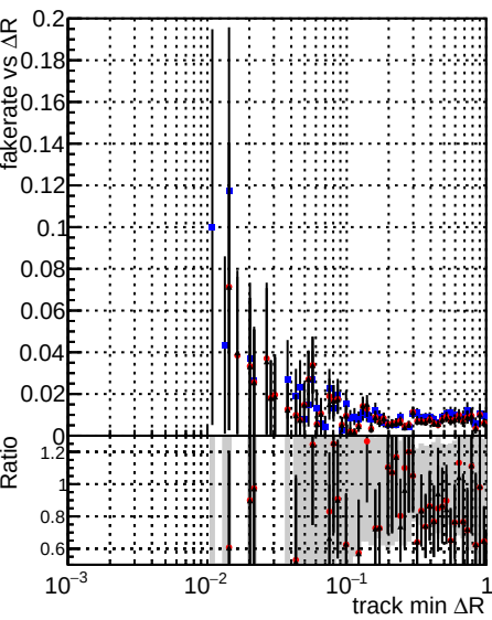
Fake rate vs \Delta R(\text{track}, \text{jet}) Legend: DQMstep3_SoftQCD_CKF (blue circles) DQMstep3_SoftQCD_default (red circles) DQMstep3_SoftQCD_ckfPixelLess (black circles)
