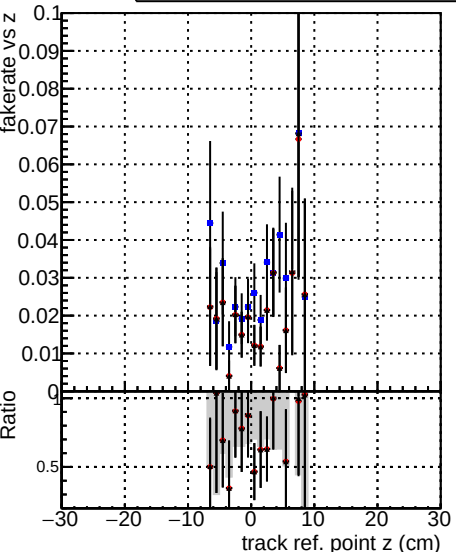
Fake rate vs verpos —•— DOMstep3_SoftQCD_CKF —•— DOMstep3_SoftQCD_default —•— DOMstep3_SoftQCD_ckfPixelLess
