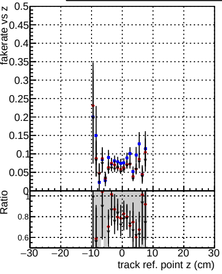
Fake rate vs verpos Legend: DQMstep3_SoftQCD_CKF (blue dots) DQMstep3_SoftQCD_default (red dots) DQMstep3_SoftQCD_ckfPixelLess (black dots)
