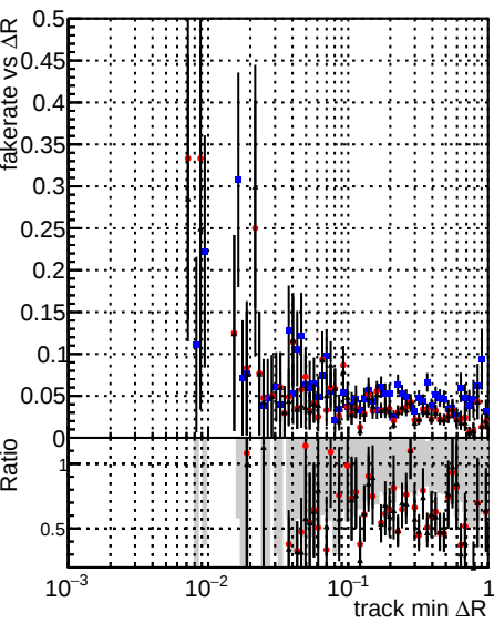
Legend: DQMstep3_SoftQCD_CKF (blue squares), DQMstep3_SoftQCD_default (red circles), DQMstep3_SoftQCD_ckfPileLess (black triangles)
