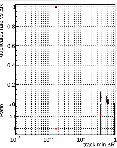
DOMstep3_SoftQCD_CKF DOMstep3_SoftQCD_default DOMstep3_SoftQCD_ckfPixelLess
