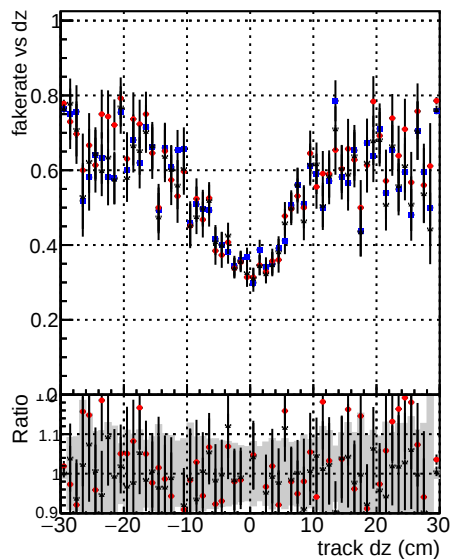
DOMstep3 SoftOCD-CKF DOMstep3 SoftOCD-CKF-PixelLess
