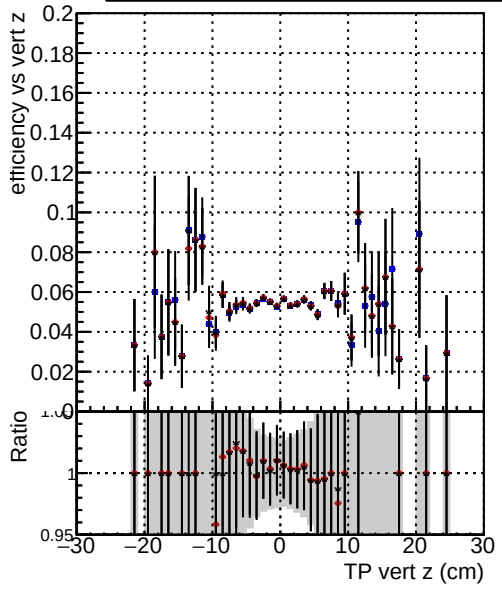
Efficiency vs. TP vert z (cm) —●— DQMstep3_SoftQCD_CKF —●— DQMstep3_SoftQCD_default —●— DQMstep3_SoftQCD_ckfPixelLess
